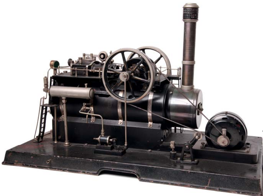
8016 Märklin, 4159/11/94 Kraftanlage, Originalzustand, großes Dampflokomobil stationär mit zwei feststehenden doppelwirkenden Zylindern und zwei Schwungräder. Mit Dynamo 3394/1, L68cm. Mit Lackschäden an Bodenplatte im Brennerbereich, ansonsten Z1-2
